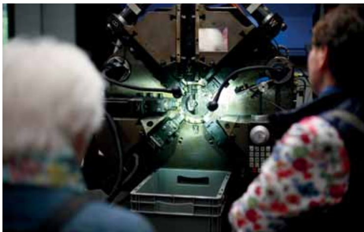
Die Biegemaschine für Titandraht. Sie wird jeden Tag manuell neu programmiert, da kein Meter Draht dem anderen zu 100% gleicht.
